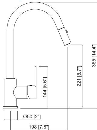
MINIMA single lever with spring pull down shower Monomando de fregadero industrial MINIMA con caño de muelle y ducha extraíble
