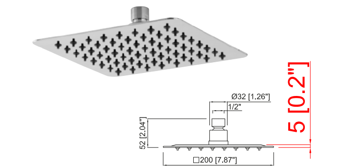
Ultra thin shower-head, 8.00" x 8.00" Rociador de ducha ultra fino de 200 x 200 mm
