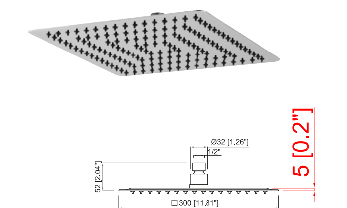
Ultra thin shower-head, 12.00" x 12.00" Rociador de ducha ultra fino de 300 x 300 mm
