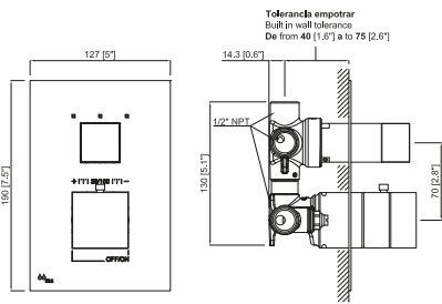
Ceramic diverter Inversor cerámico
