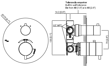
Brass solid flange Plafón sólido de latón
