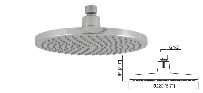
Shower-head Ø9.00" Rociador de ducha de Ø220 mm
