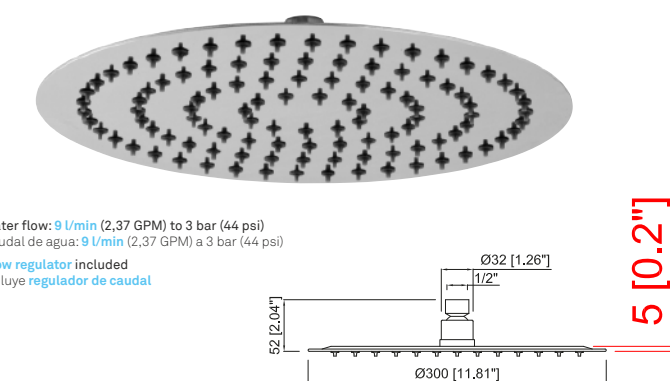
Ultra thin shower-head Ø12.00" Rociador de ducha ultra fino Ø300 mm
