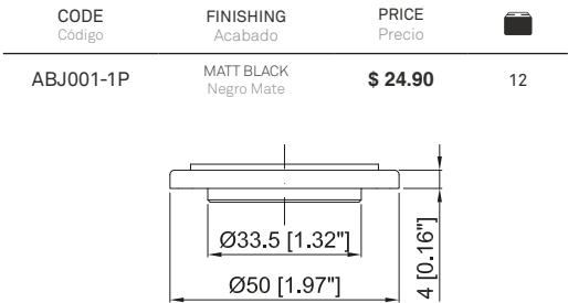
Base plate for a better installation in sinks with wide holes Aro base para una mejor instalación en lavabos con agujeros fuera de medidas
