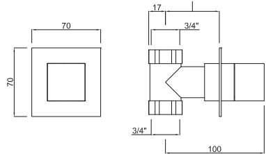
Ceramic setting Montura cerámica
