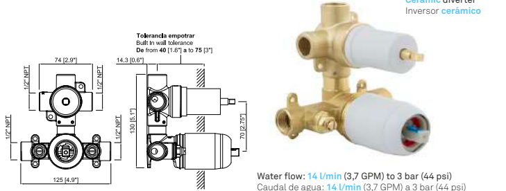
CMB023-1K Ceramic diverter Inversor cerámico
