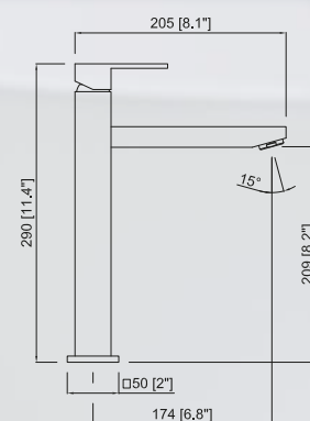
Single lever lavatory with high 6.8" spout Monomando de lavabo alto con caño de 17 cm
