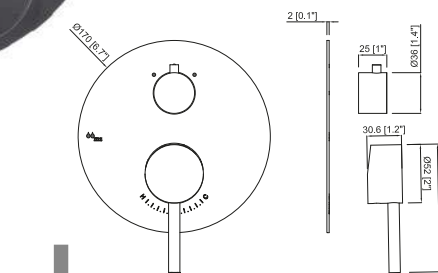
Ceramic diverter Inversor cerámico
