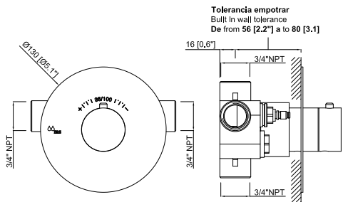
Brass solid flange Plafón sólido de latón
