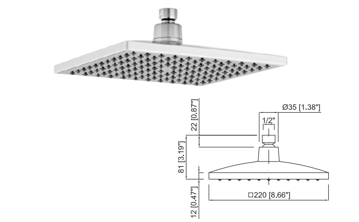
Shower-head 9.00" x 9.00" Rociador de ducha de 220 x 220 mm
