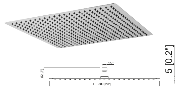
Ultra thin shower-head 20,00" x 20,00" Rociador de ducha ultra fino de 500 x 500 mm
