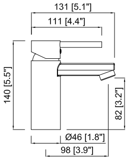
Single lever bidet Monomando de bidé
