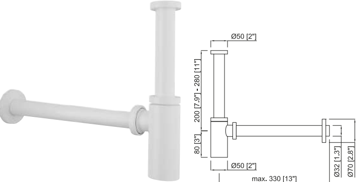
Minimalist trap Sifón minimalista
