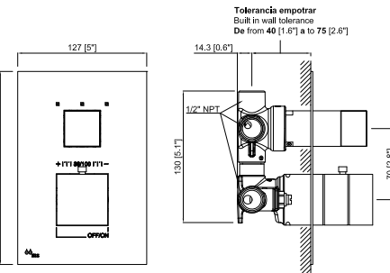
Brass solid flange Plafón sólido de latón
