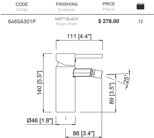
Single lever bidet Monomando de bidé
