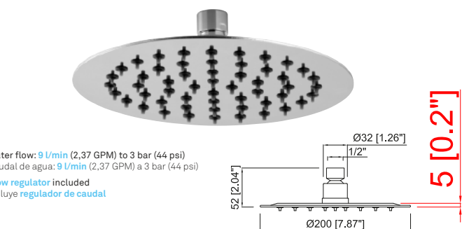
Ultra thin shower-head Ø8.00" Rociador de ducha ultra fino Ø200 mm
